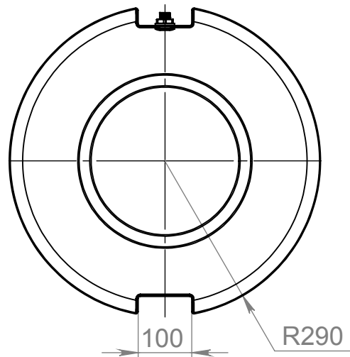
В-В (1 : 10)
